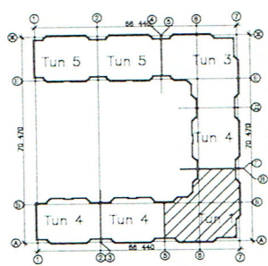
Схема блокировки
